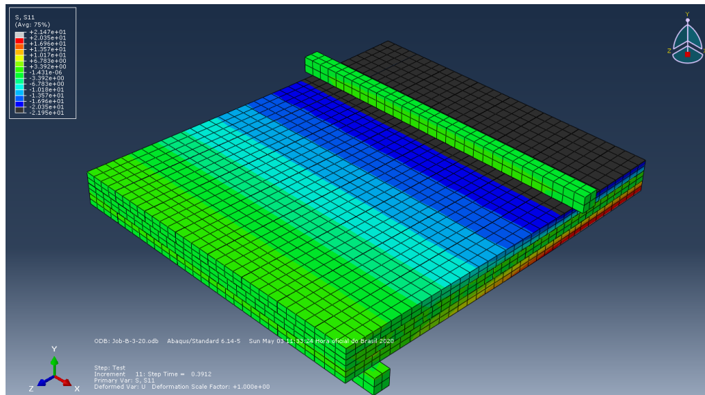
Figura 6.29 – Tensão de escoamento alcançada com uma força de 34,7 kN
