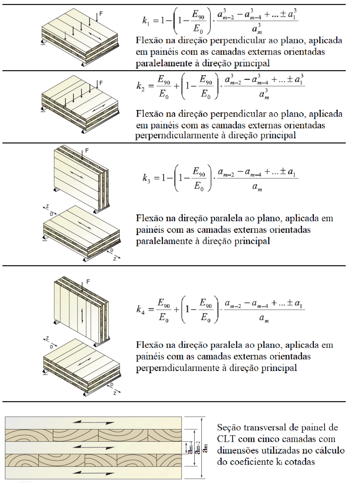
Figura 3.4 – Diferentes situações de carregamento previstas pelo k-Method e equações correspondentes para o cálculo do coeficiente k_i
