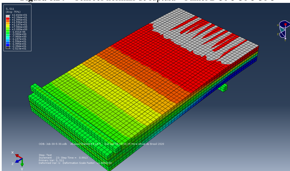
Figura 6.24 – Tensões normais de ruptura – Painel B-30-5-30-5-30-5
