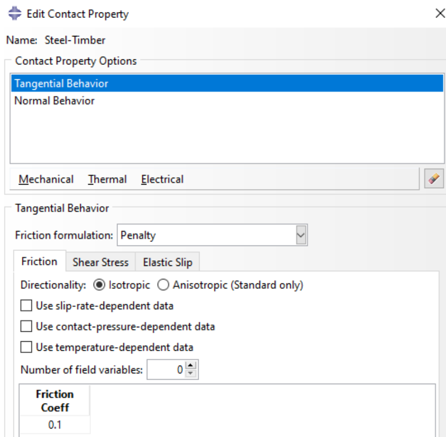
Figura 5.9 – Propriedade de interação atribuída ao contato entre as peças de aço e as de madeira
