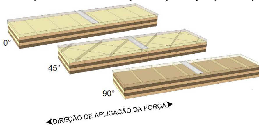
Figura 2.22 – Configurações geométricas dos painéis ensaiados com diferentes orientações das camadas em relação à direção de aplicação da força
