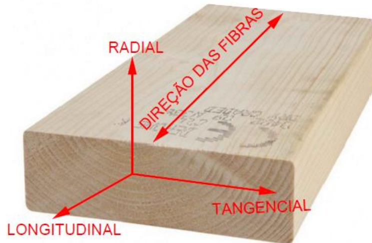
Figura 4.2 – Orientações de interesse para a análise das propriedades mecânicas da madeira
