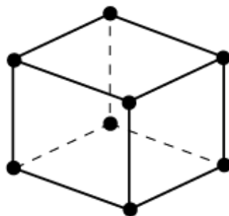
Figura 5.6 – Elemento C3D8
