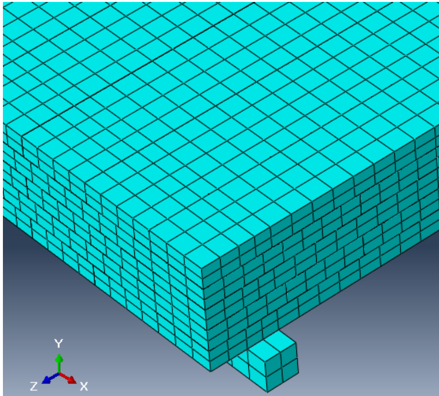
Figura 5.7 – Malha adotada em uma das modelagens
